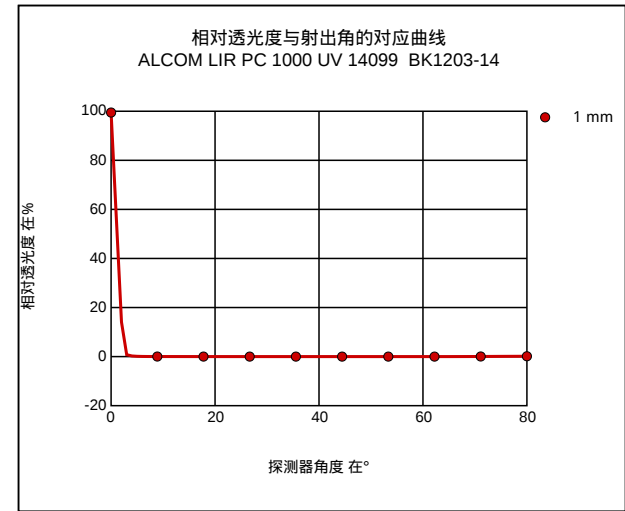
相对透光度与射出角的对应曲线
