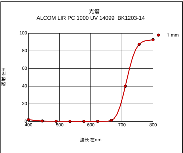
光谱
